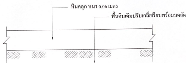
รายละเอียดถนนหินคลุก Not Scale
